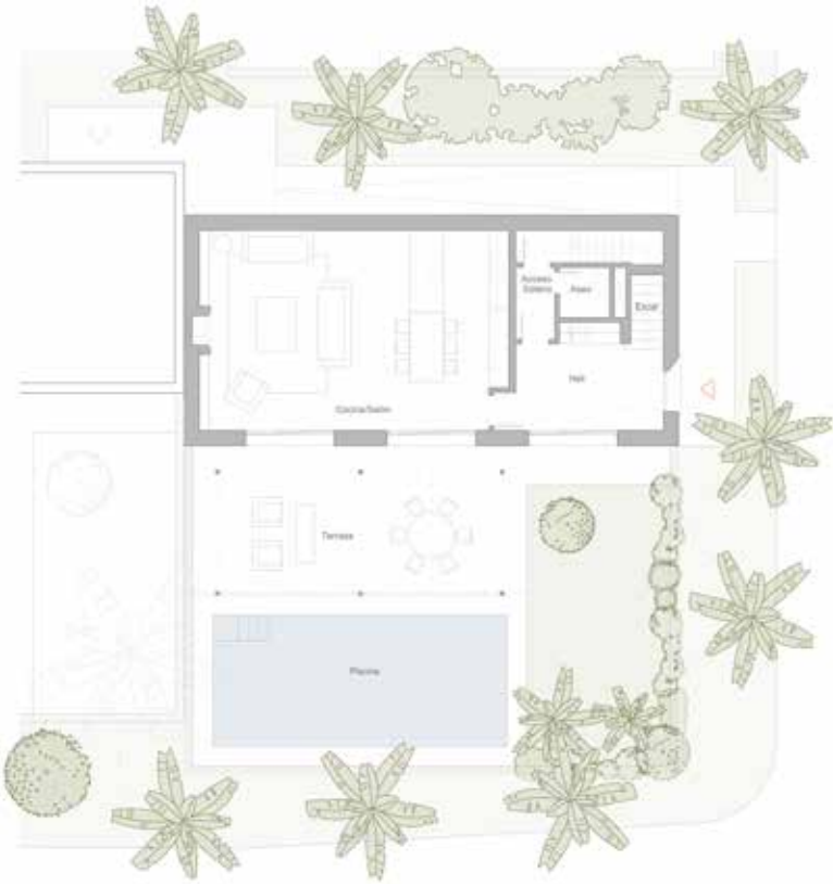
Planta Baja
