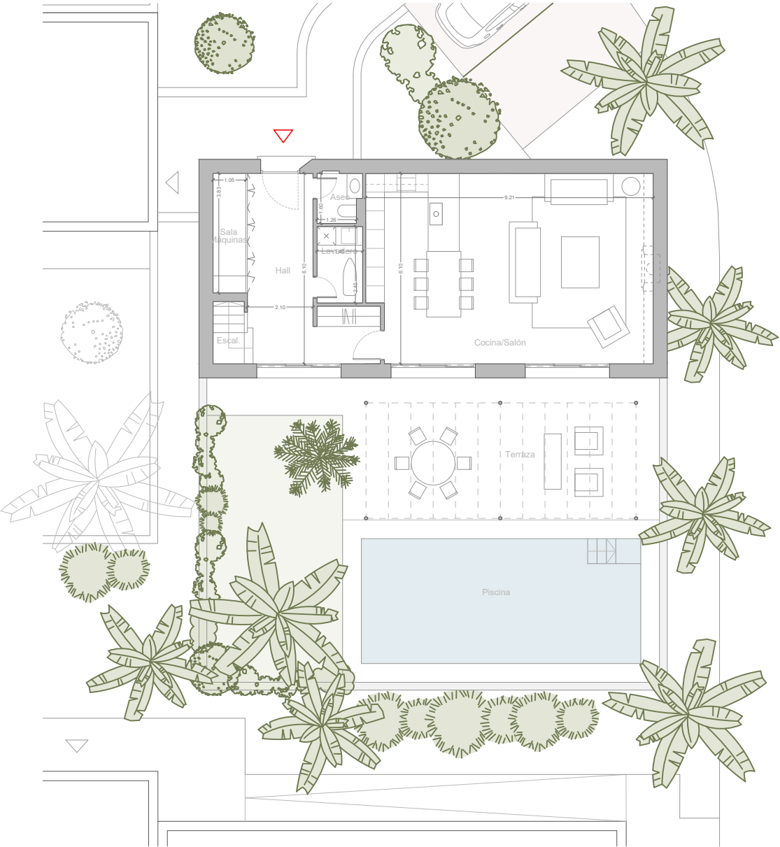
Planta Baja
