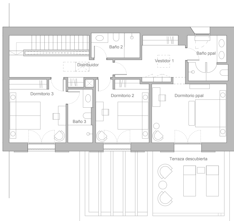
Planta Primera
