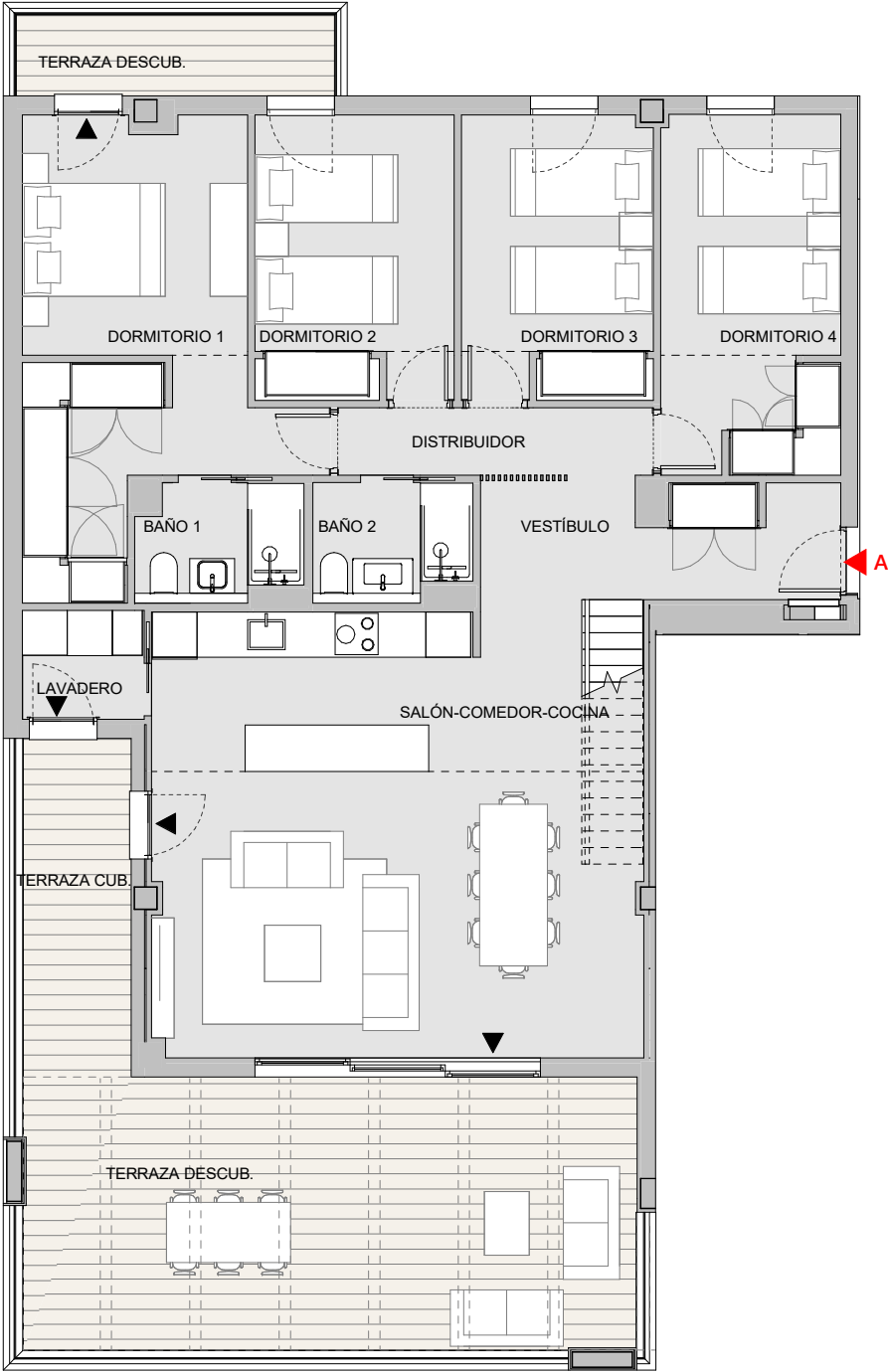
Planta segunda
