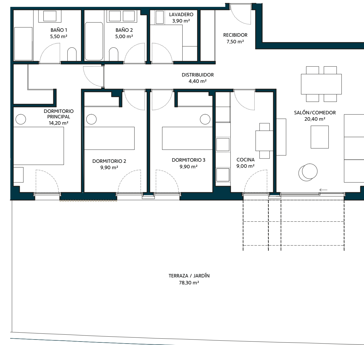
PLANTA BAJA CON ZONAS EXTERIORES
